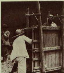
Los hombres de los Andes venezolanos trabajan con esmero y cuidado en la fabricación de las tapias con que han de levantar sus viviendas. El modo de hacer las tapias es sumamente sencillo: basta con echar la tierra en una horma y apisonarla luego. Las tapias son muy resistentes.
