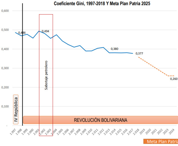
Gráfico 2 Coeficiente Gini
