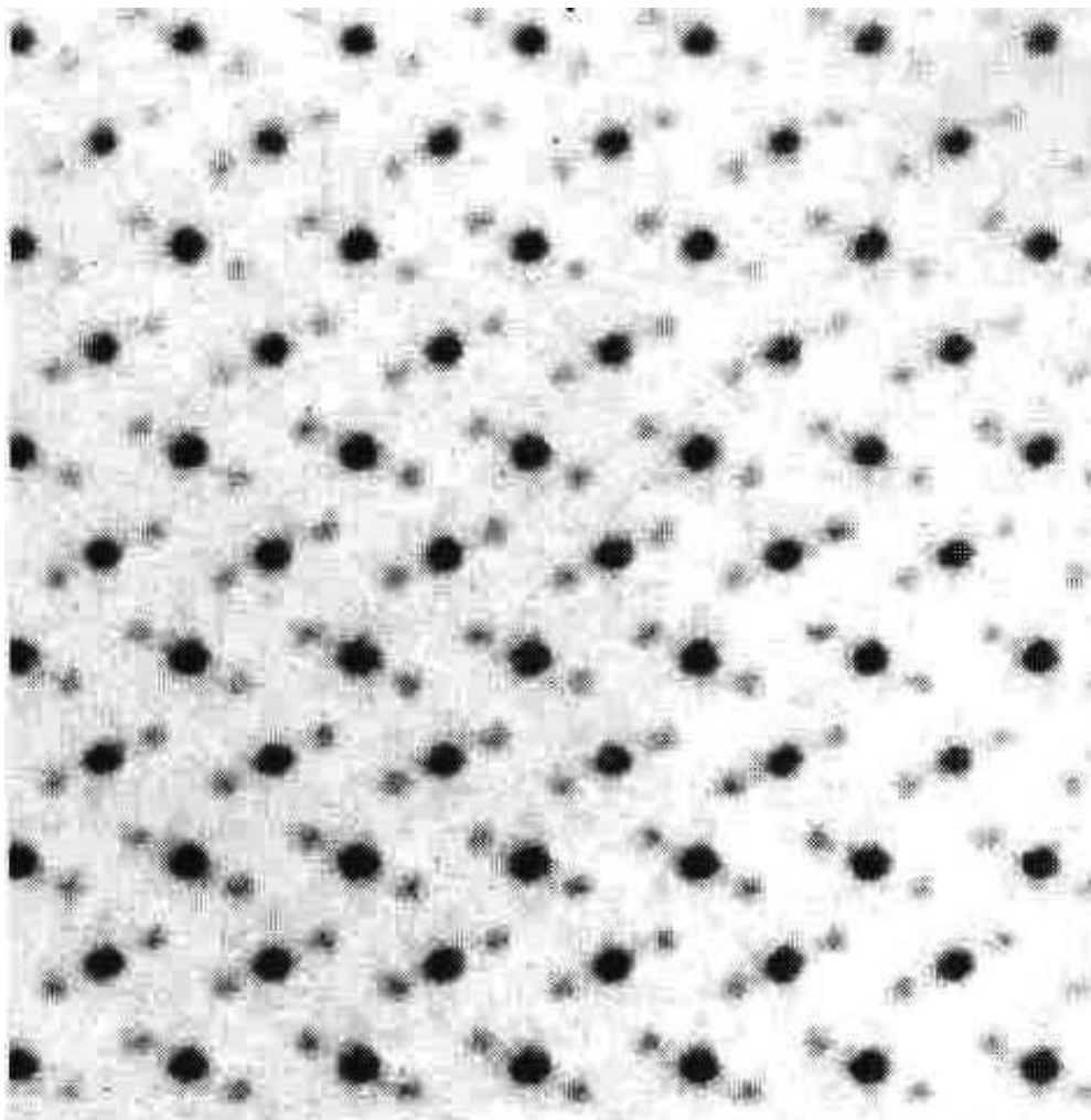
Átomos del mineral marcasita, aumentados 4.5 millones de veces con un microscopio que utiliza luz visible y rayos X. La marcasita es un cristal donde se repite la unidad FeS 2 : Fe indica hierro y está representado por las manchas grandes, S indica azufre y está representado por los pares de puntos pequeños que flanquean cada átomo de hierro. (Cedida por el Instituto Profesor Martin J. Buerger, Instituto de Tecnología de Massachussets.
