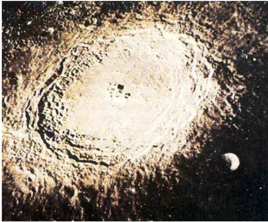
Amanecer en el cráter Copérnico, exactamente al norte del ecuador lunar. Tiene 100 kilómetros de diámetro. Cuando, a diferencia de esta fotografía, el cráter está iluminado de cara, su sistema de rayos destaca mucho. Foto del vehículo orbital Apolo. (Cedida por la NASA. )
