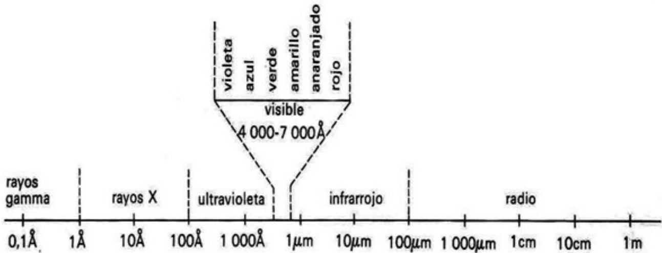
Diagrama esquemático del espectro electromagnético, desde la longitud de onda más corta (rayos gamma) hasta la más larga (ondas de radio). La longitud de onda de la luz se calcula en Angstroms (Å), micrómetros (μm), centímetros (cm) y metros (m)
