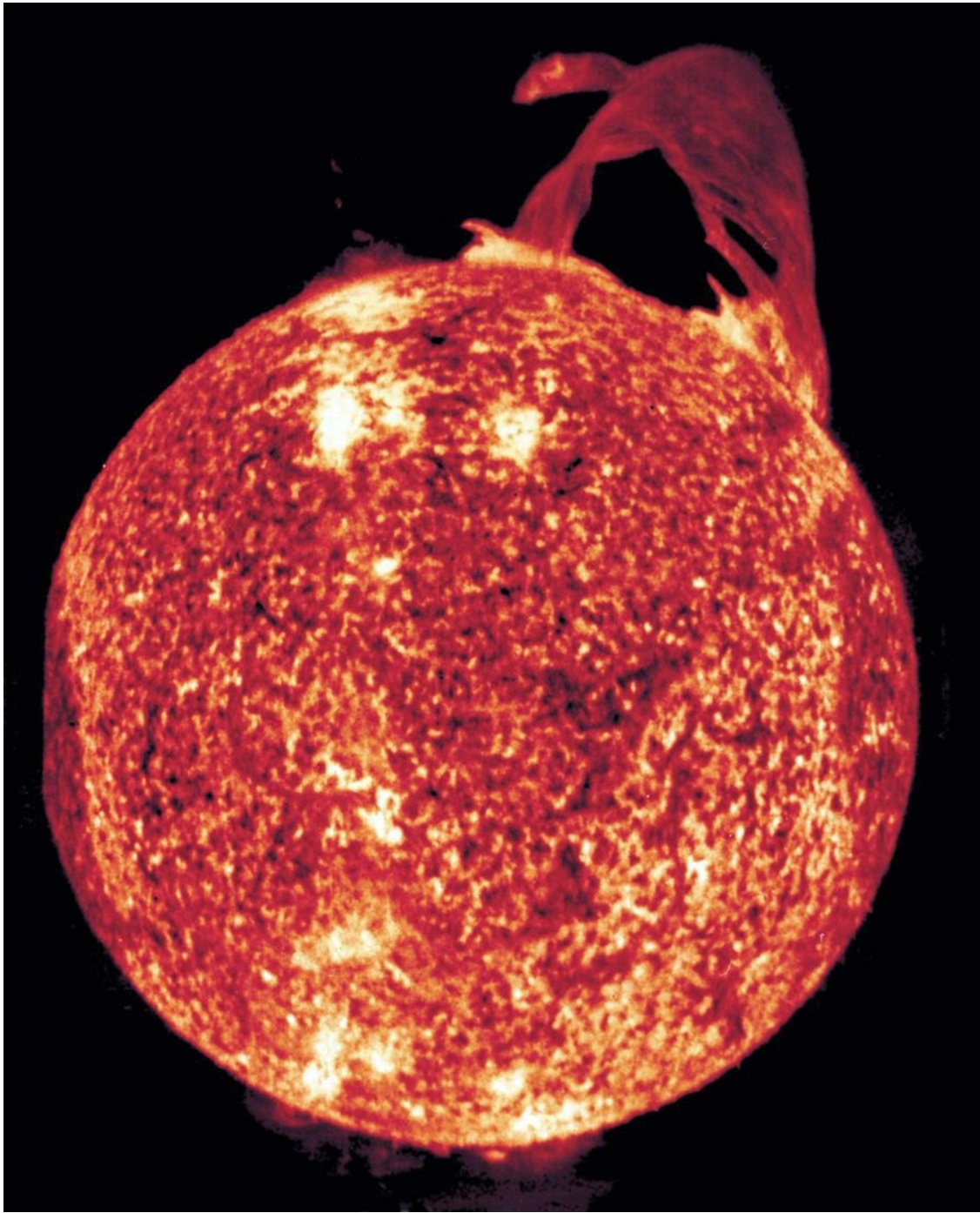
La estrella más cercana: el Sol visto a la luz de helio ionizado en el ultravioleta lejano. La prominencia solar que se proyecta arriba a la derecha se extiende momentáneamente unos 300 000 kilómetros dentro del espacio hasta que vuelve a caer sobre el gas ardiente que es la superficie visible del Sol. Las manchas más pequeñas de gas caliente visibles en esta imagen de la superficie solar tienen aproximadamente el tamaño de la Tierra. Fotografía del Skylab 4. (Cedida por la NASA.)
