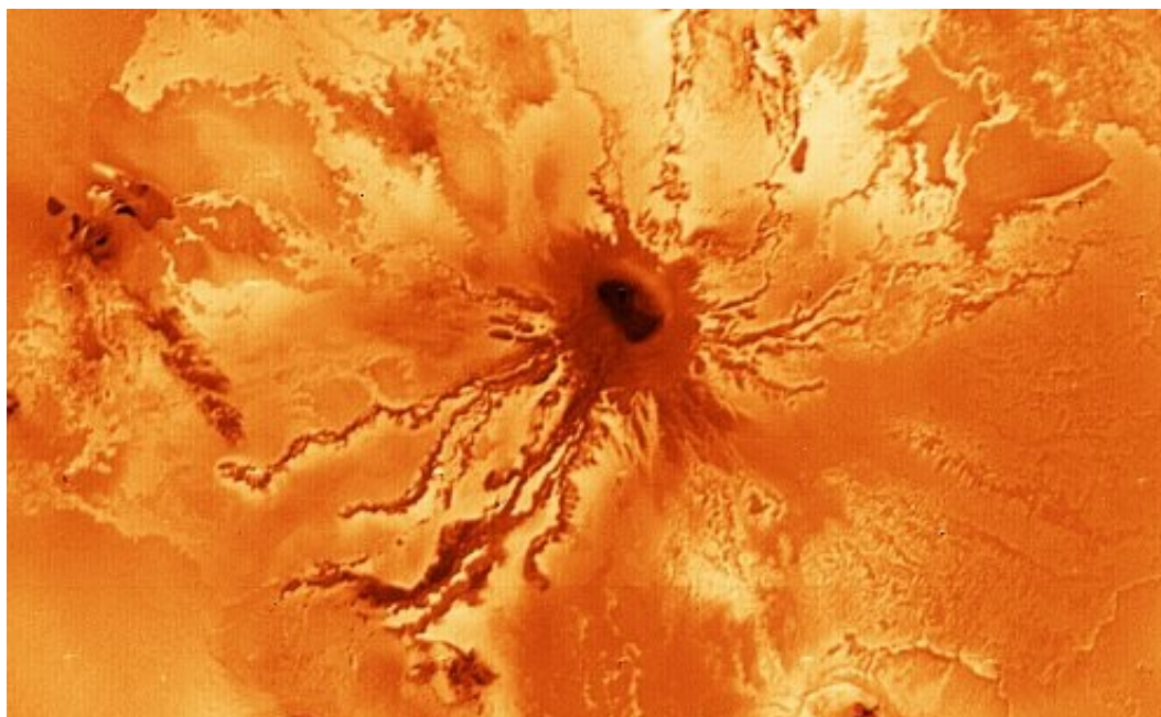
Corrientes recientes de azufre fundido procedentes del volcán Ra Patera en Io. Estamos contemplando casi directamente desde arriba la caldera volcánica. Imagen del Voyager 1. (Cedida por la NASA.)
