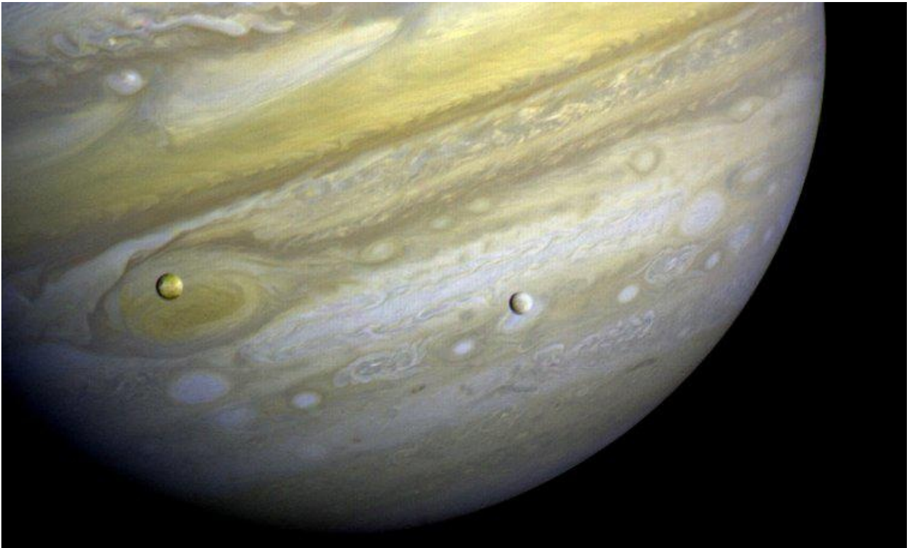
El Voyager se acerca a Júpiter, con las dos lunas Io y Europa en primer plano. (Cedida por la NASA.)
