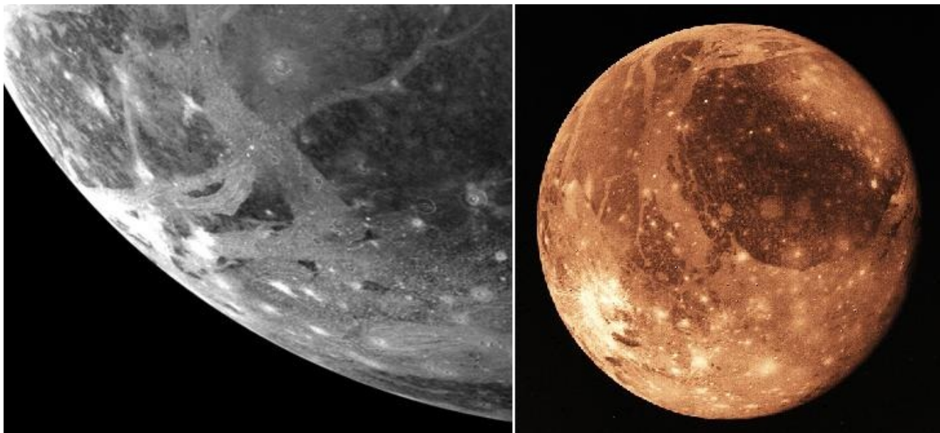
Ganímedes, la mayor luna de Júpiter. Los rasgos visibles más pequeños de esta imagen (izquierda) del Voyager tienen unos tres kilómetros de diámetro. Destacan numerosos cráteres de impacto, muchos con rayos brillantes. Las bandas que se tuercen suavemente y se cortan están compuestas de surcos paralelos de origen incierto, (Cedida por la NASA.)
