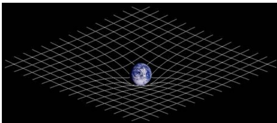
Representación esquemática de la distorsión de un espacio plano por un objeto de gran masa.
