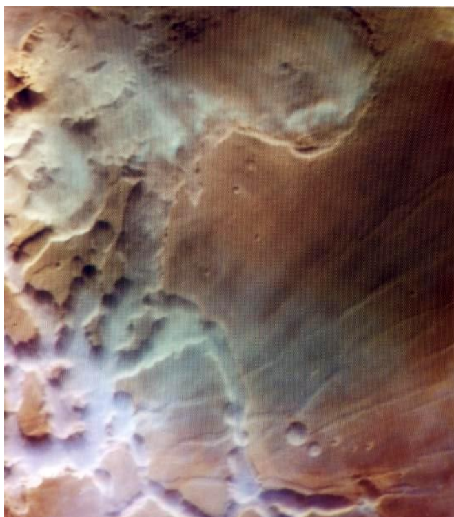
Neblina matutina y escarcha en el terreno profundamente erosionado de Noctis Labyrinthus, Laberinto de la Noche. Foto del vehículo orbital Viking. (Cedida por la NASA.)
