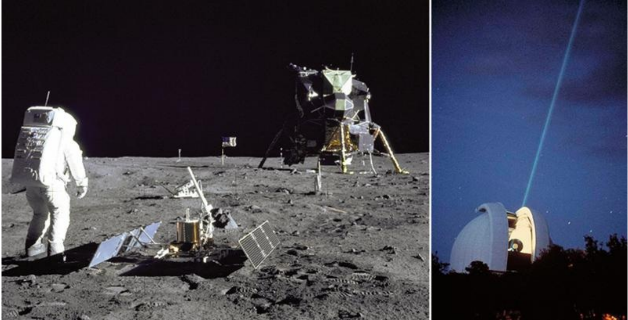
Astronautas del Apolo 16 instalan el experimento de un retrorreflector de láser en la Luna (izquierda). (Cedida por la NASA.) Rayo láser dirigido a los retrorreflectores situados en la superficie lunar. El telescopio es el reflector de 82 pulgadas del observatorio McDonald, Universidad de Texas (derecha).
