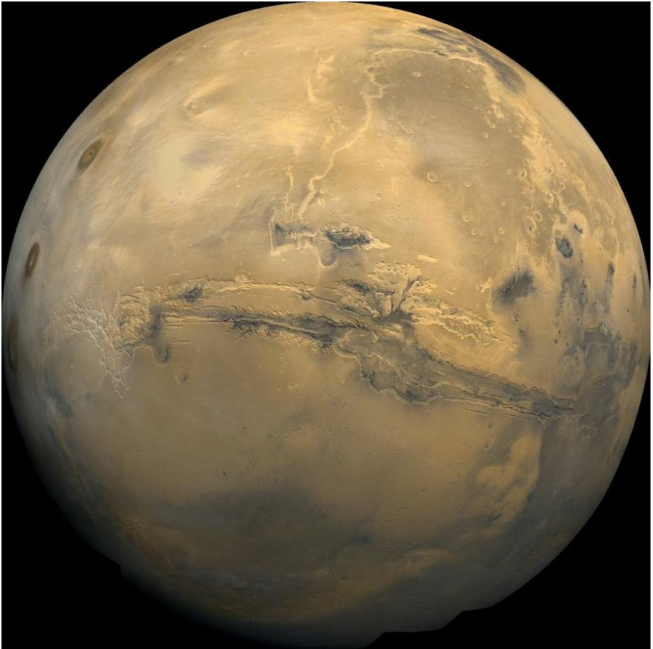
Mosaico de Marte, compuesto por más de 100 imágenes obtenidas por el orbitador Viking (NASA/JPL)
