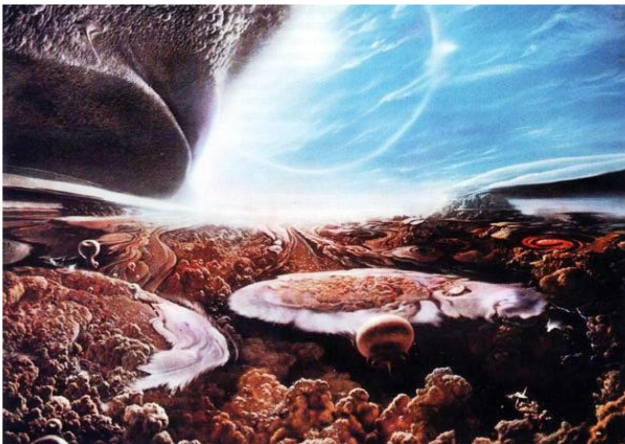
Cazadores y flotantes, formas vivas imaginarias pero posibles en la atmósfera de un planeta de tipo joviano. Las formas de las nubes son en su mayoría las que el Voyager descubrió en Júpiter. Los cristales de hielo en la alta atmósfera causan el halo alrededor del Sol. (Pintura de Adolf Schaller.)
