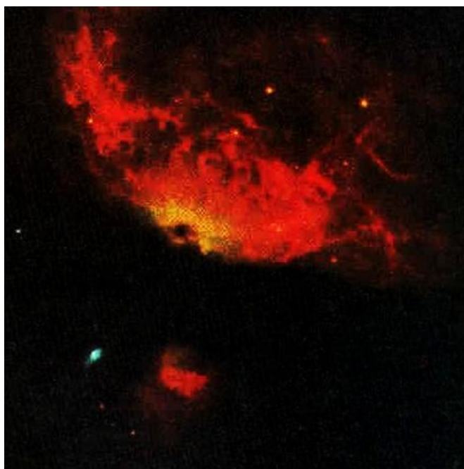
Una excursión al interior de la Gran Nebulosa de Orión. El gas, estimulado por la luz de estrellas calientes, brilla con varios colores. Parte de la nebulosa está oscurecida por una nube de polvo absorbente. La Nebulosa de Orión puede verse a simple vista desde la tierra.
