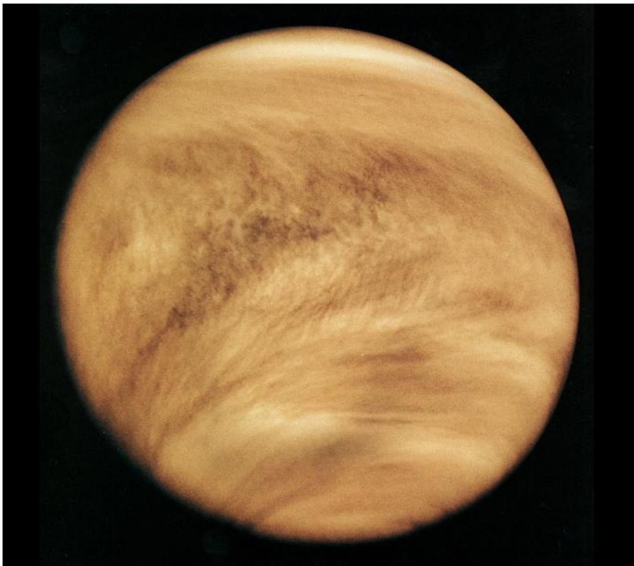
El disco entero de Venus en luz ultravioleta, impreso en los tonos del espectro visible. Las formas se deben a las nubes, que giran de derecha a izquierda, en la alta atmósfera de Venus. Foto del vehículo orbital Pioneer Venus. (Cedida por la NASA.)
