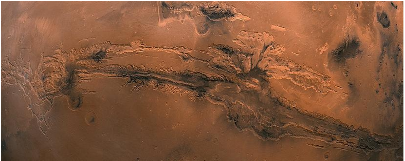
El gran Valle del Mariner, Vallis Marineris. Descubierta por el Mariner 9 en 1971-1972, tiene 5 000 kilómetros de longitud y aproximadamente 100 kilómetros de ancho. Se ven valles afluentes causados posiblemente por corrientes de agua y rayas dibujadas por el viento, relacionadas con cráteres de impacto. (NASA)
