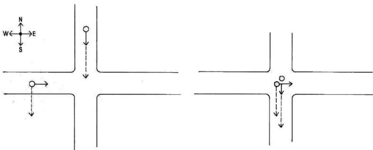
La paradoja de la simultaneidad en relatividad especial. El observador está mirando desde el brazo meridional de un cruce. Un ciclista se acerca desde el norte a una velocidad indicada por la flecha de trazo continuo. La luz reflejada por el ciclista se acerca al observador a una velocidad más alta, indicada por la flecha de trazos. Un coche se acerca al cruce desde el oeste a una velocidad indicada por la flecha de trazo continuo, y una luz se refleja de él hacia el ser a una velocidad dada por la correspondiente flecha de trazos. Si fuera correcto sumar la velocidad del ciclista a la velocidad de la luz (puesto que el ciclista se aproxima al observador), la luz
