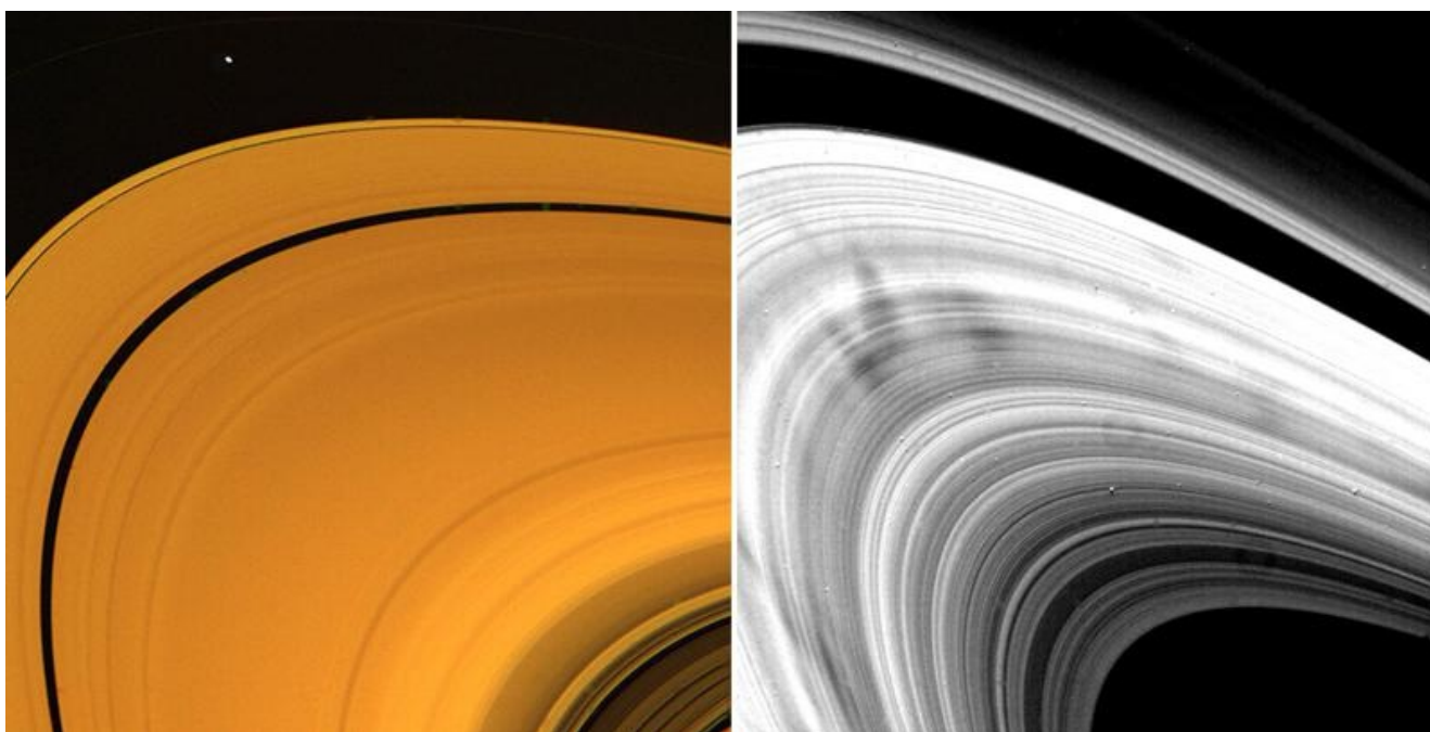
Imágenes de los anillos de Saturno, obtenidas por el Voyager 2 (NASA/JPL.)
