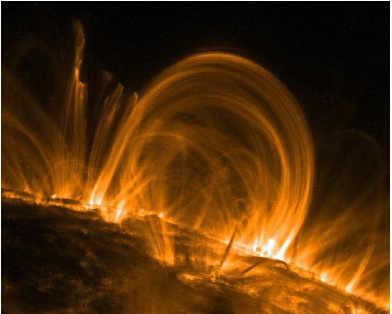
Bucles de gas caliente e ionizado sobre una región solar activa que se ven obligados a seguir las líneas de fuerza magnética locales, como las limaduras de hierro en el campo de un imán (NASA/TRACE)
