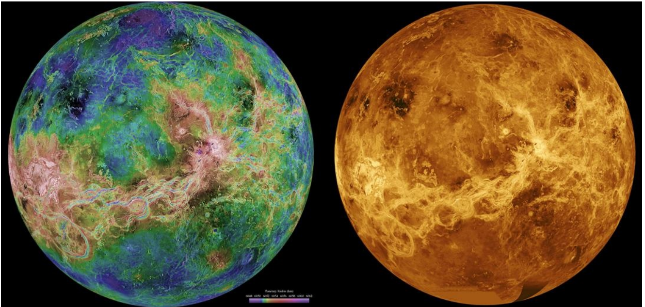
Mapa por radar de la superficie de Venus, obtenido la por mision Magallanes de 1990-1994 (NASA/JPL/USGS)
