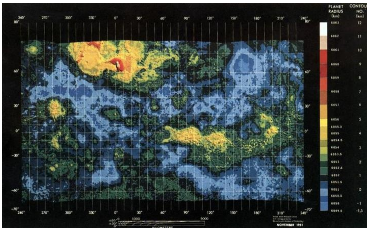
Mapa topográfico de Venus obtenido por la Pioneer. En la parte superior la Ishtar Terra y los Montes Maxwell (NASA)
