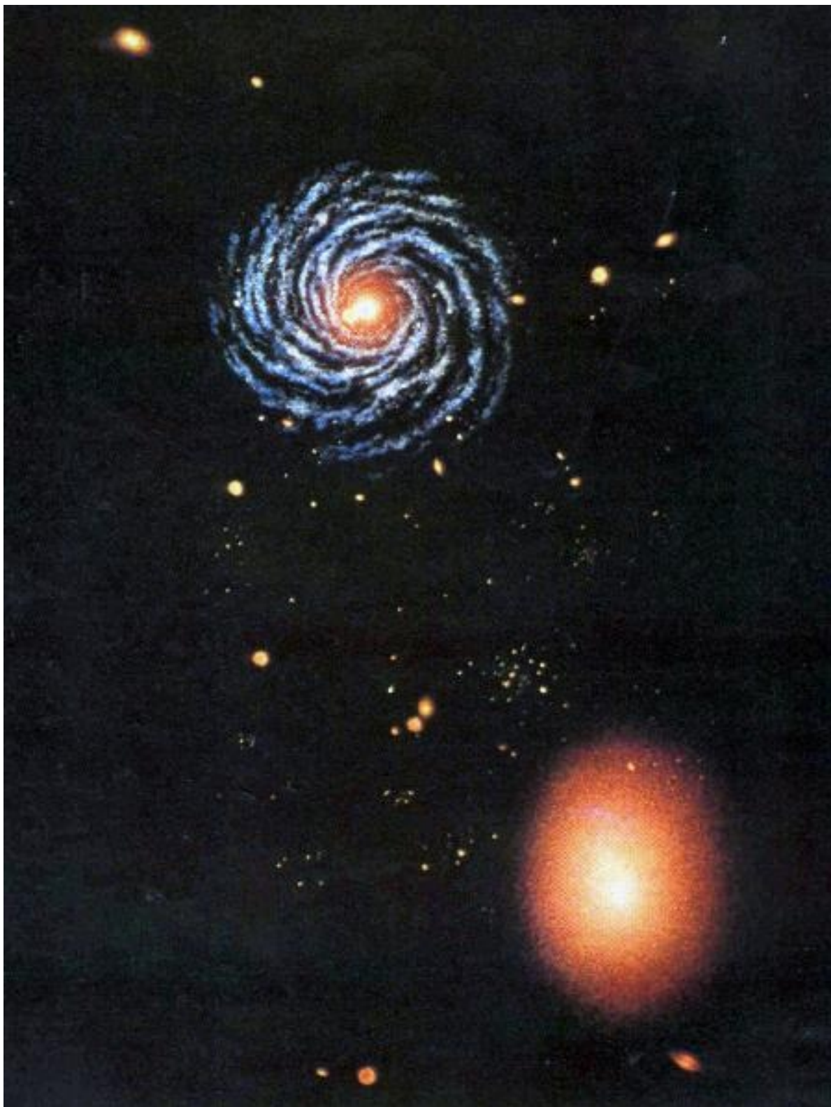
Un quasar en el interior de una galaxia elíptica gigante dominando un cúmulo profuso de galaxias. (Pintura de Adolf Schaller.)
