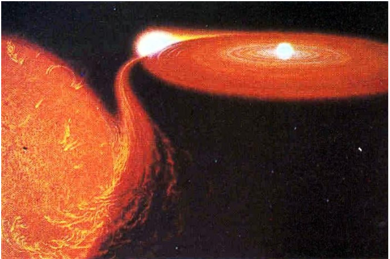
Fases posteriores de la evolución estelar. La atmósfera estelar luminosa de una binaria de contacto fluye de la estrella gigante roja (izquierda) al disco de acreción alrededor de una estrella pulsar de neutrones (derecha). El disco brilla en rayos X y otras radiaciones en el punto de contacto. (Pintura de Don Davis.)
