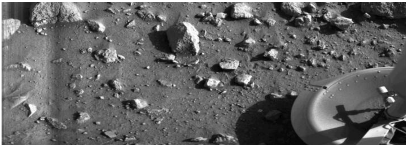
La primera imagen de la superficie de Marte que haya llegado a la Tierra, radiada el 20 de julio de 1976. A la derecha se observa parte del pie de aterrizaje número 2, asentado de modo seguro sobre la superficie. Más tarde se descubrió que otro pie de aterrizaje estaba enterrado en la arena. La roca vesicular del centro tiene unos diez centímetros de diámetro
