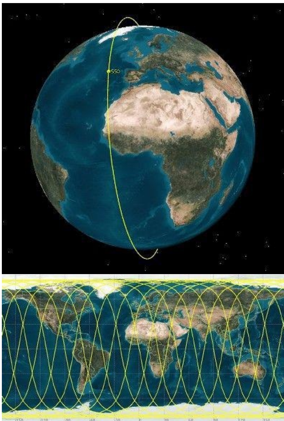
Imágenes: Vista tridimensional y traza terrestre de una órbita heliosíncrona, a veces también denominada polar por su paso cercano a los polos terrestres. Ampliamente utilizada por satélites de observación terrestre. (Imagen:
