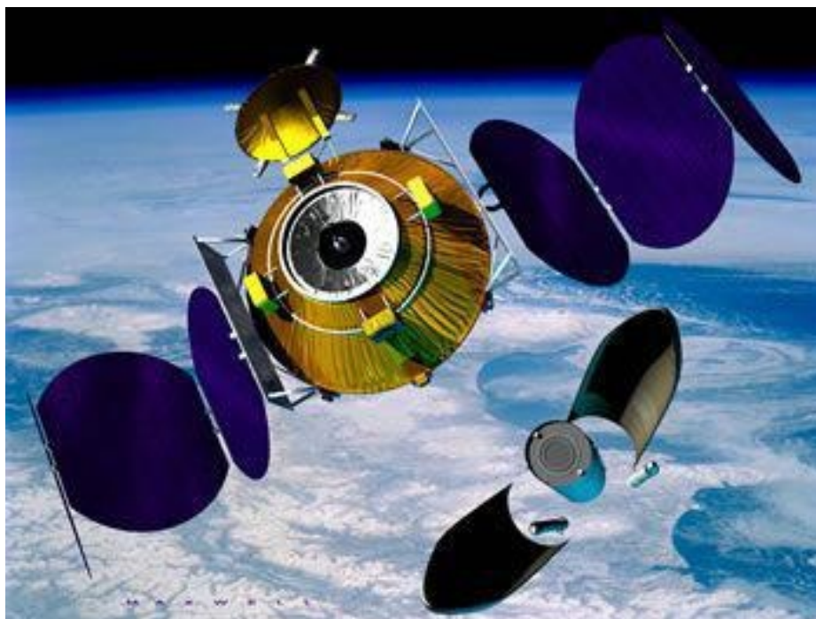
Imagen: ConeXpress utiliza la estructura cónica del adaptador de carga útil del Ariane 5 como parte principal de su estructura, de modo que no ocupa ningún espacio adicional a bordo del lanzador. (Imagen: Orbital Recovery Ltd )
