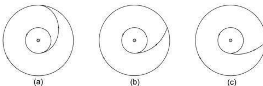
Imagen: Tres tipos de órbitas de transferencia entre órbitas circulares coplanarias: a) órbita de Hohmann, la más lenta y económica; b) órbita de transferencia tangente a la órbita inicial, la mejor opción después de la de Hohmann en cuanto a economía; c) órbita no tangente a la órbita inicial ni a la final: la menos económica pero más rápida. (Esquema: J.Casado)
