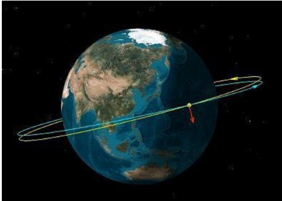
Imagen: Efectos de arrojar un objeto con una velocidad reducida respecto a la del vehículo espacial, de forma lateral con respecto a la dirección de desplazamiento. En amarillo, la órbita de partida (vehículo); en azul, la órbita obtenida (objeto arrojado). Efecto exagerado para mayor claridad. (Imagen: J.Casado)
