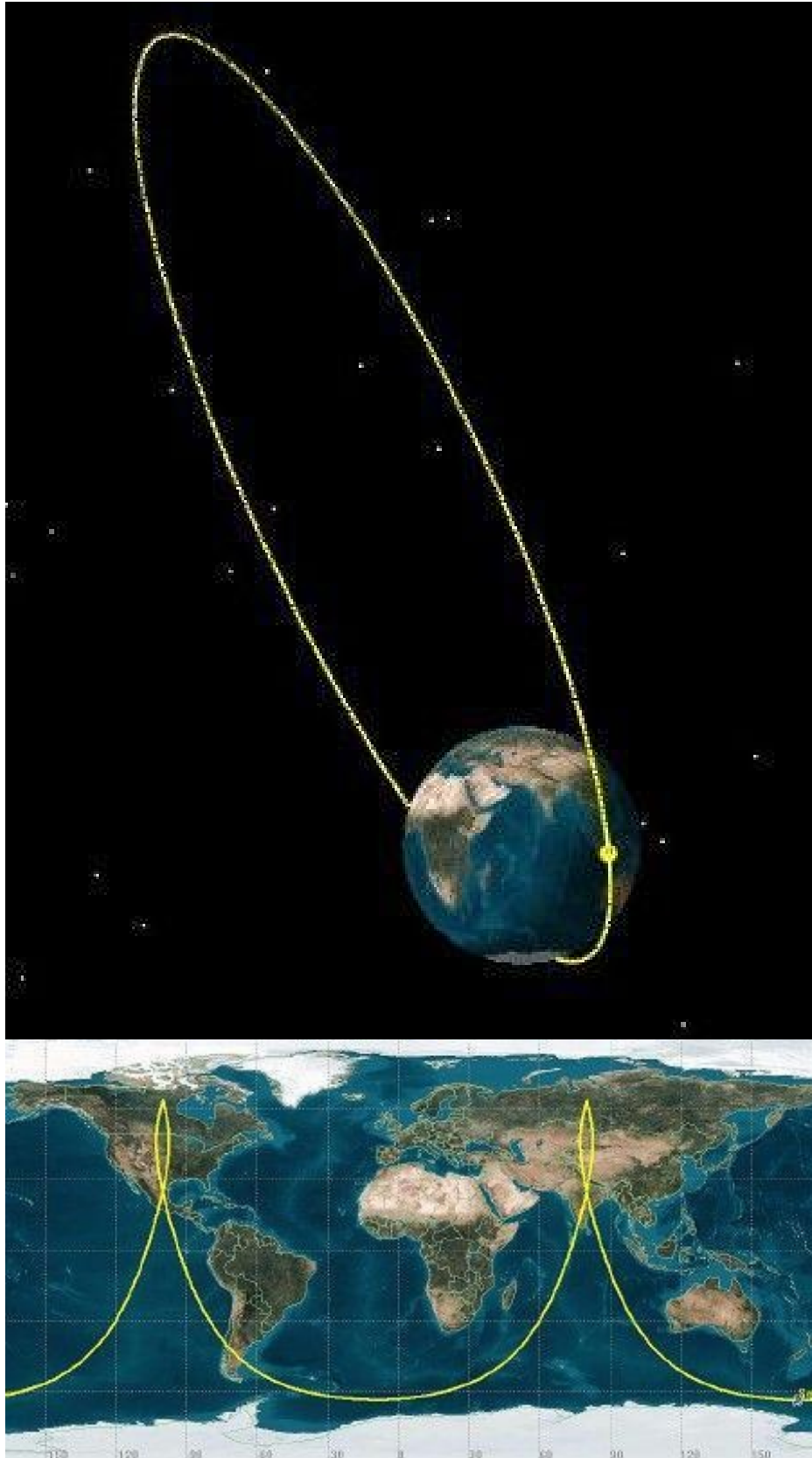
Imágenes: Vista tridimensional y traza terrestre de una órbita Molniya, utilizada principalmente por satélites de comunicaciones rusos. (Imagen: J.Casado)
