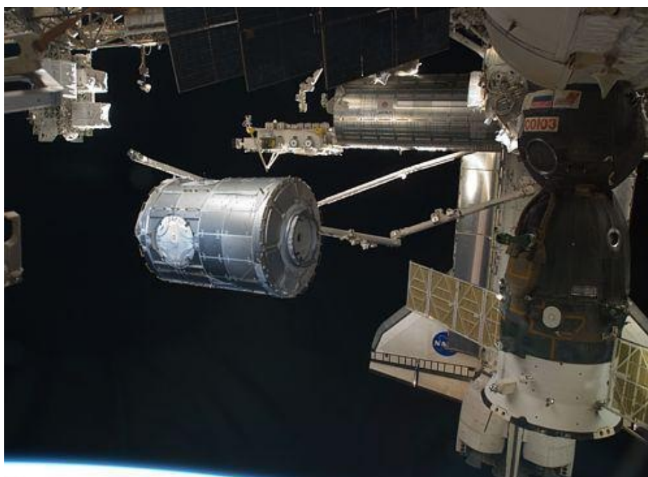
Imagen: El Nodo 3, bautizado como “Tranquility”, en el proceso de su acoplamiento a la Estación Espacial Internacional el 12 de febrero de 2010. Sobre él se instalaría poco después la cúpula. A la derecha, en primer plano, una nave Soyuz acoplada a la estación. (Foto: NASA)
