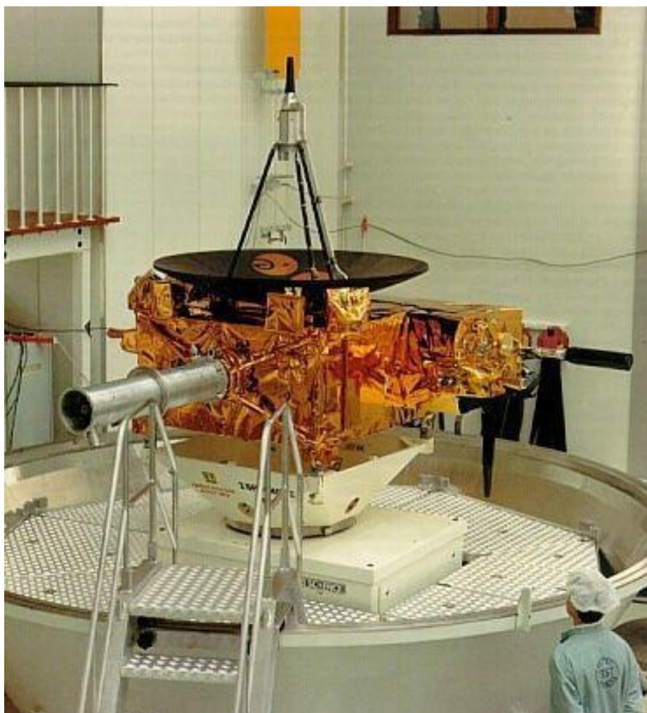
Imagen: El recubrimiento dorado de buena parte de satélites y sondas espaciales corresponde a las mantas térmicas que aíslan al vehículo del medio ambiente espacial. (Foto: ESA)
