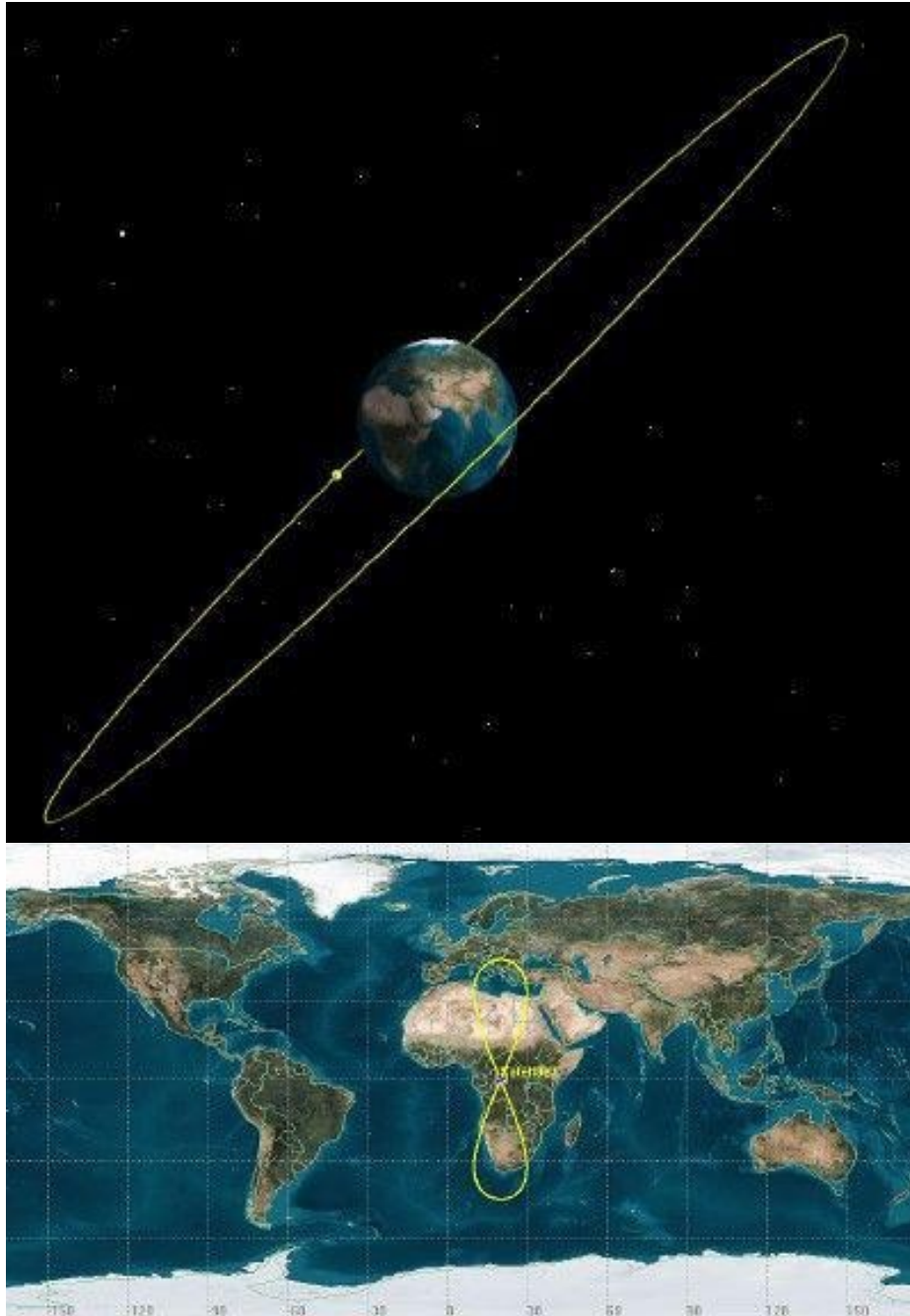
Imágenes: Vista tridimensional y traza terrestre de una órbita geosíncrona circular de inclinación 45^\circ . (Esquema: J.Casado)
