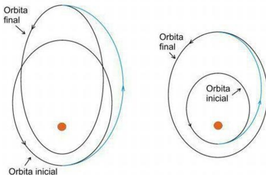
Imagen: En el caso de transferencia entre una órbita circular y otra elíptica (ambas coplanarias), la órbita más económica es la que conecta el mayor apocentro con el pericentro de la otra órbita. (Esquema: J.Casado)
