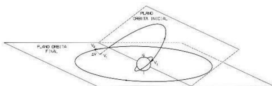
Imagen: Transferencia típica de órbita de aparcamiento a órbita geoestacionaria (caso particular de transferencia entre órbitas circulares no coplanarias). La órbita inicial tiene su inclinación mínima limitada por la latitud del lugar de lanzamiento, obteniéndose dicha inclinación mínima con un lanzamiento hacia el este; para lograr la órbita geoestacionaria de inclinación 0^\circ se requiere, por tanto, un cambio de órbita posterior. El cambio de plano orbital se deja para el punto de intersección con la órbita final, consiguiéndose así una mayor economía de combustible. (Esquema: J.Casado)
