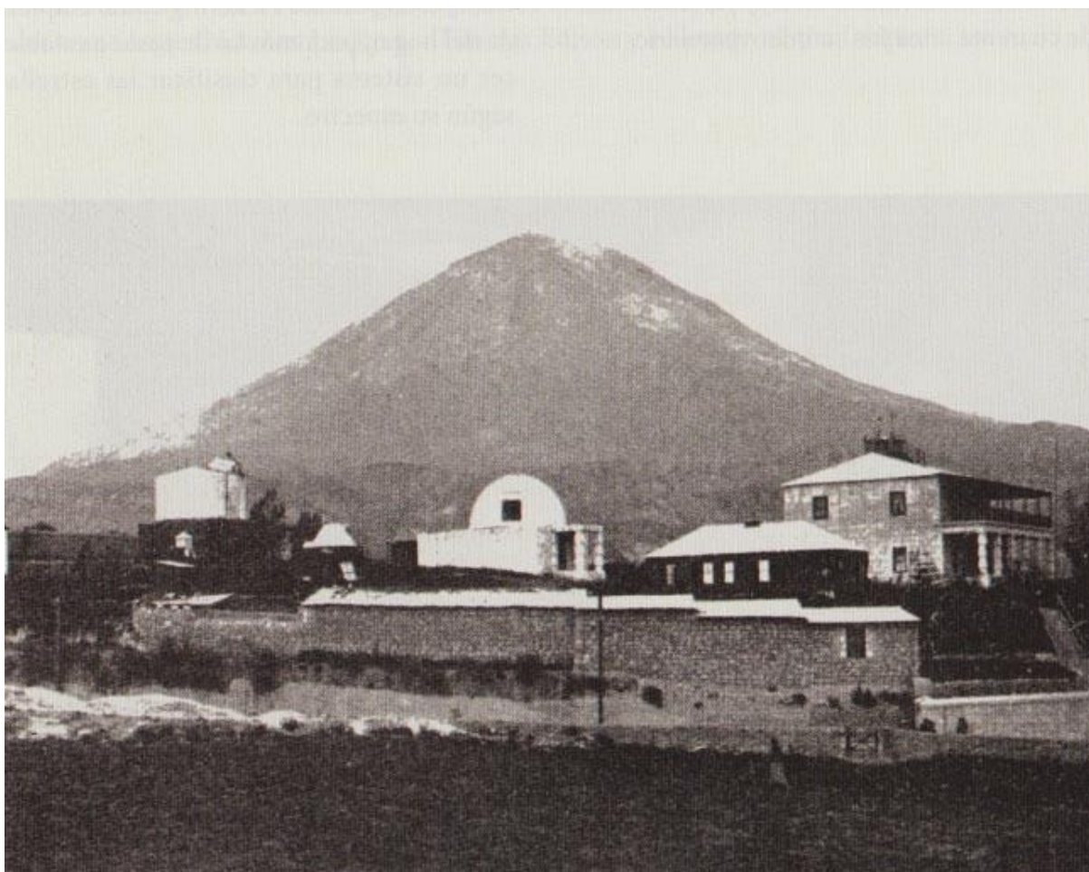
Para fotografiar las estrellas del hemisferio sur, Harvard estableció un observatorio auxiliar, la Estación Boyden, en Arequipa, Perú, teniendo a la vista el Misti, un volcán inactivo. La casa del observador construida por William Pickering está a la derecha.
