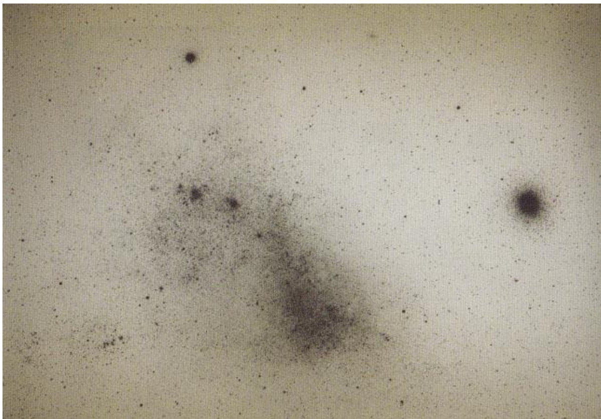
Las estrellas aparecen como puntos oscuros en este negativo de la Pequeña Nube de Magallanes, una galaxia satélite de la Vía Láctea que se puede observar desde el hemisferio sur. La mancha de la derecha es el cúmulo globular de estrellas conocido como 47 Tucanae.
