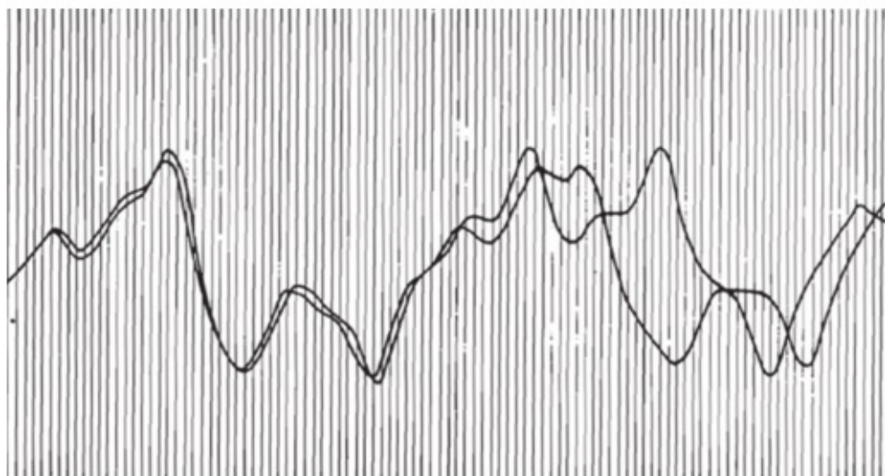
Computadora Royal McBee LGP-30 como la usada por Lorenz (arriba) y series de predicciones de Lorenz, que coinciden al principio, pero van divergiendo a medida que transcurre el tiempo (imagen de los archivos de Lorenz de 1961).
