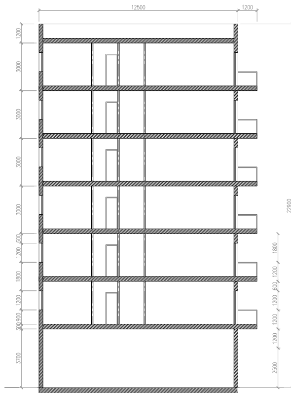
Sección transversal
