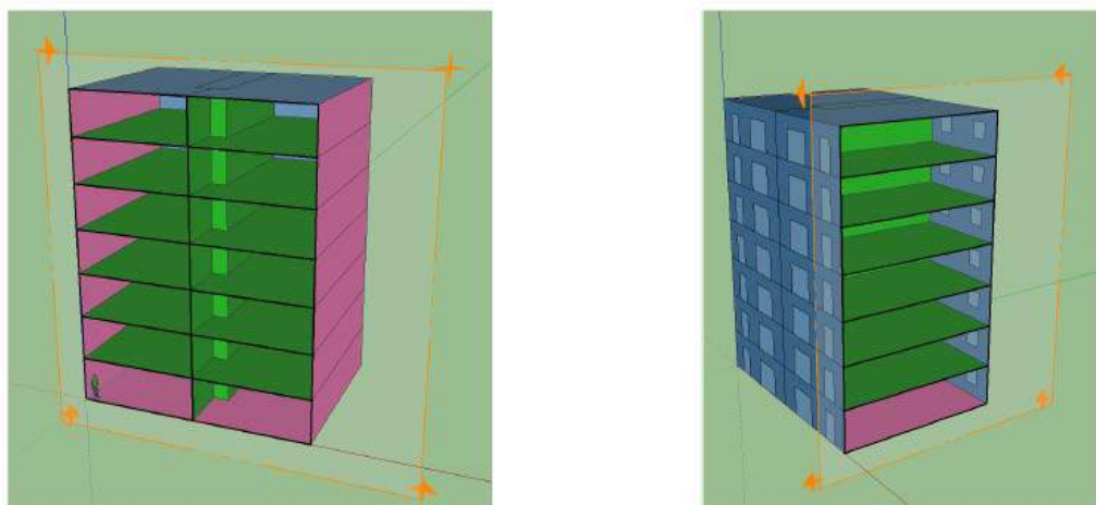
Vista 3D del edificio tipo modelado
