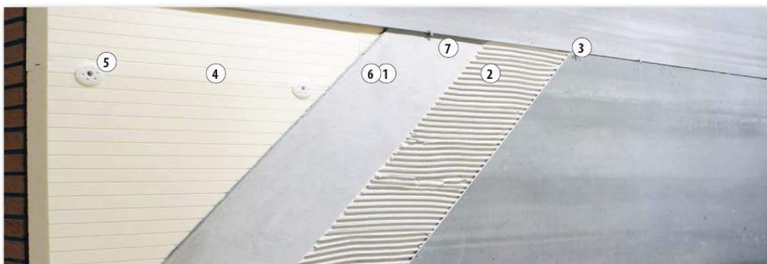
Componentes del sistema SATE cerámico de Butech. Porcelanosa
