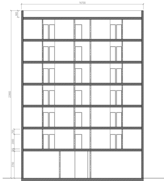
Sección longitudinal
