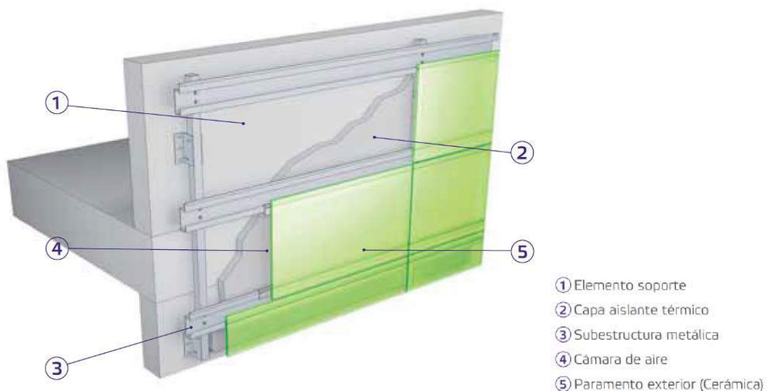
Componentes Fachada Ventilada. Fuente "fachadas ventiladas y pavimentos técnicos"
